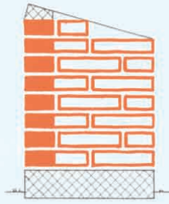
Snit, mål 1:20
