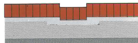
Figur 2. Afløbsrende i gangbelægning.
