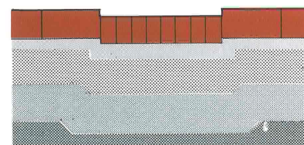
Figur 3. Afløbsrende i kørebelægning, lægges evt. i beton.
