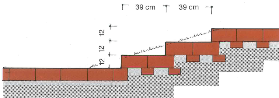
Snit i trappe, sten på kant
