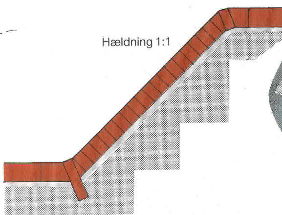
Snit i skråning, sten på kant.
