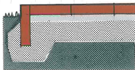
Figur 8. Sten på fladen, afsluttet med kopskifte på kant, stilles evt. i beton.
