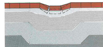
Figur 4. Afløbsrende i kørebelægning udføres som nedrundning i belægningen, lægges evt. i beton.
