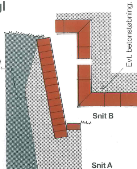
Opstalt af skrå mur, smig = 20°
