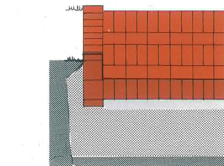
Snit B. Den underliggende sten på fladen må kun trækkes ca. 2 cm tilbage.
